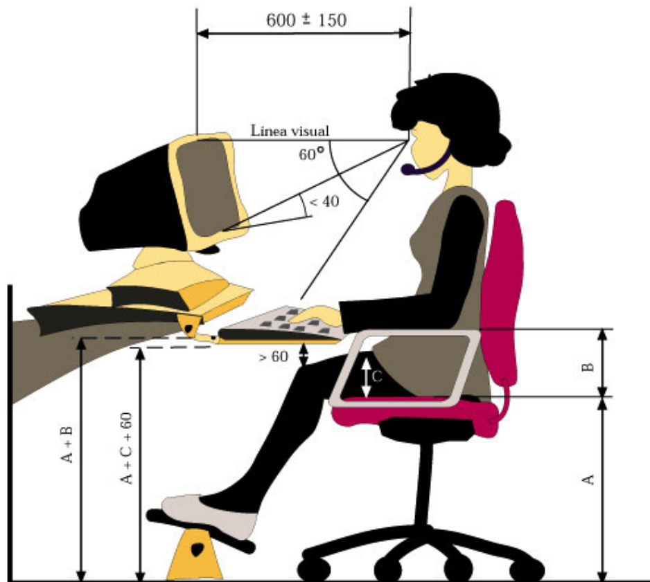
Dimensiones en milímetros
